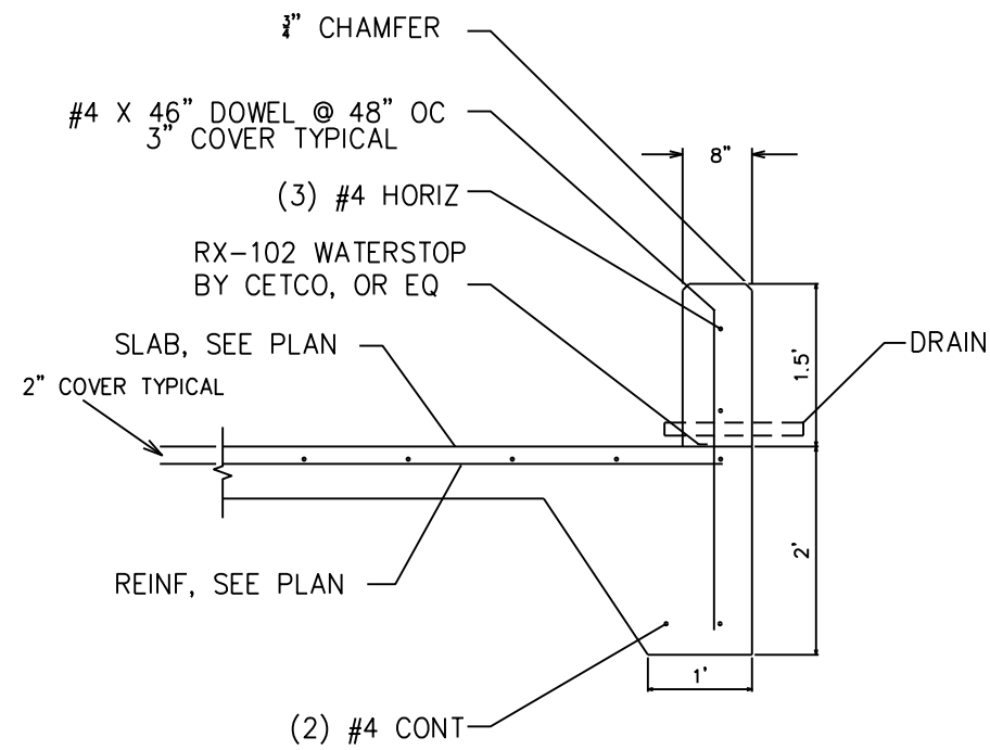
2 EXTERIOR SLAB EDGE S1 SCALE: 1" = 2'-0"
