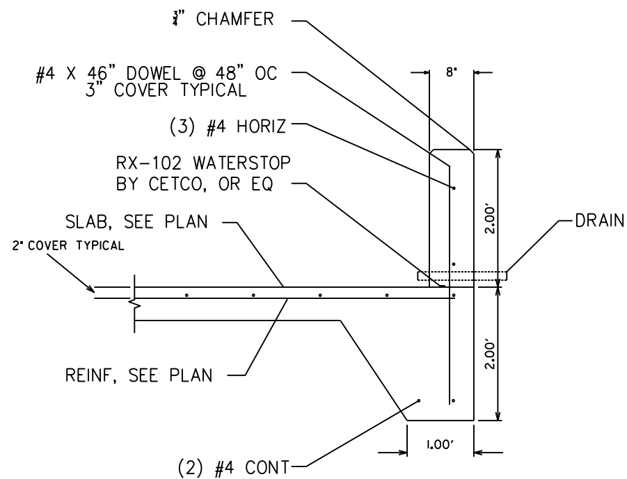
2 EXTERIOR SLAB EDGE S1 SCALE: 1/2" = 1'-0"
